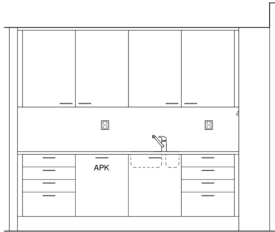
K4A 1 : 25
