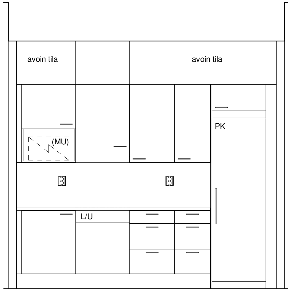
K1A 1 : 25
