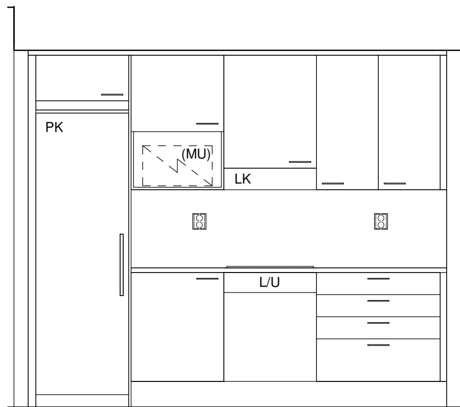
K5A 1 : 25
