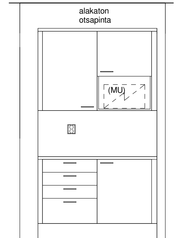
K7B 1 : 25
