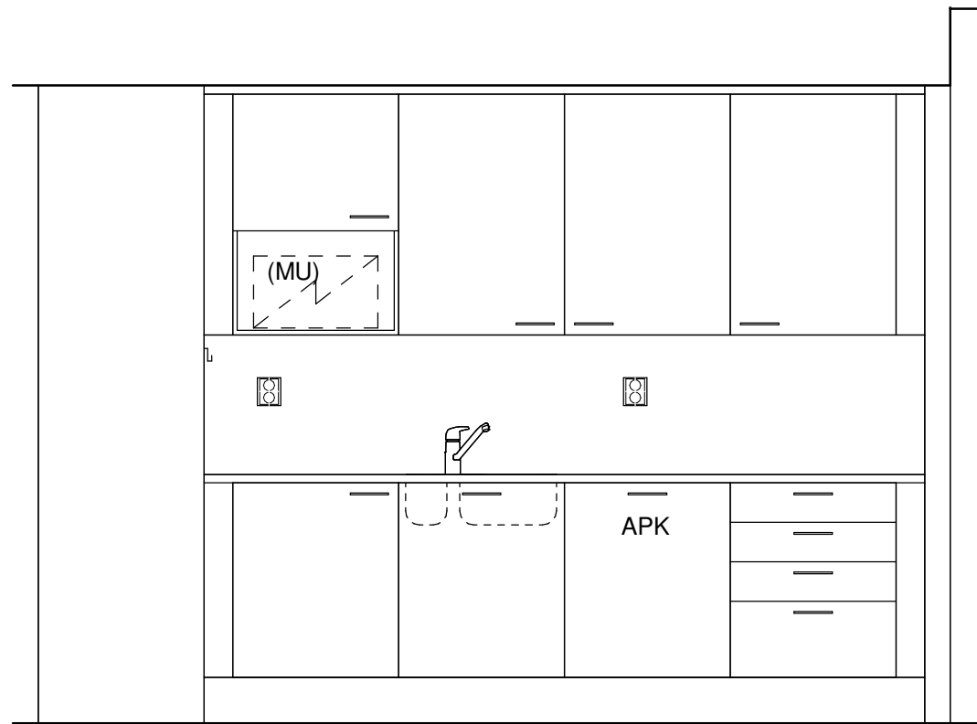
K8A 1 : 25
