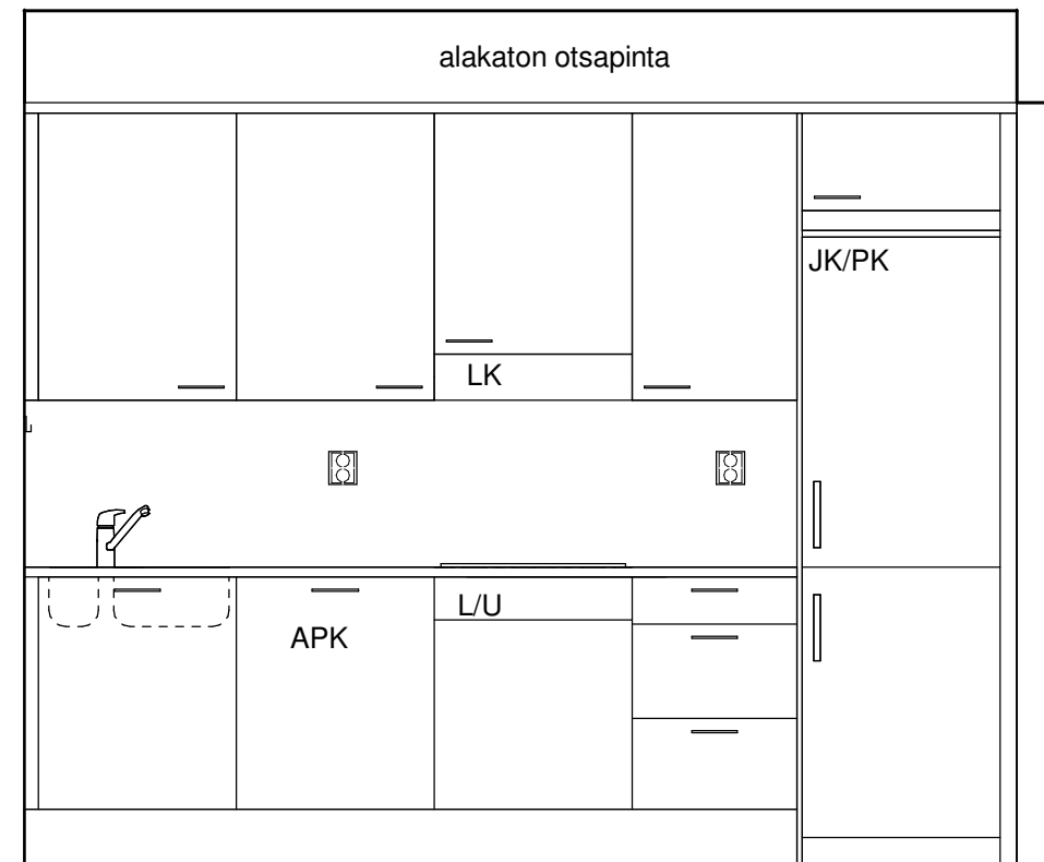
K7A 1 : 25
