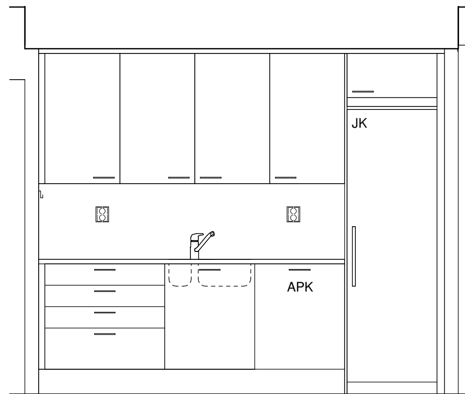
K5B 1 : 25
