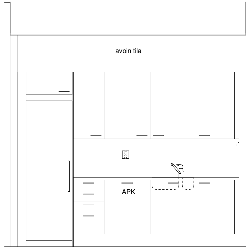
K1B 1 : 25
