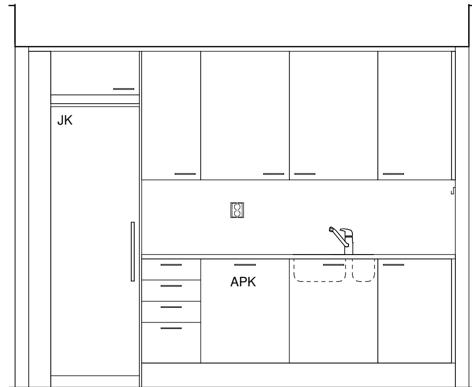
K1B 1 : 25
