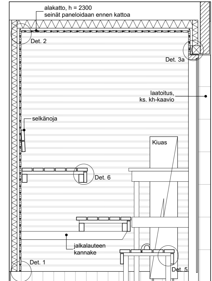
Saumot kohdakkain lattialaatoituksen saumojen kanssa!
