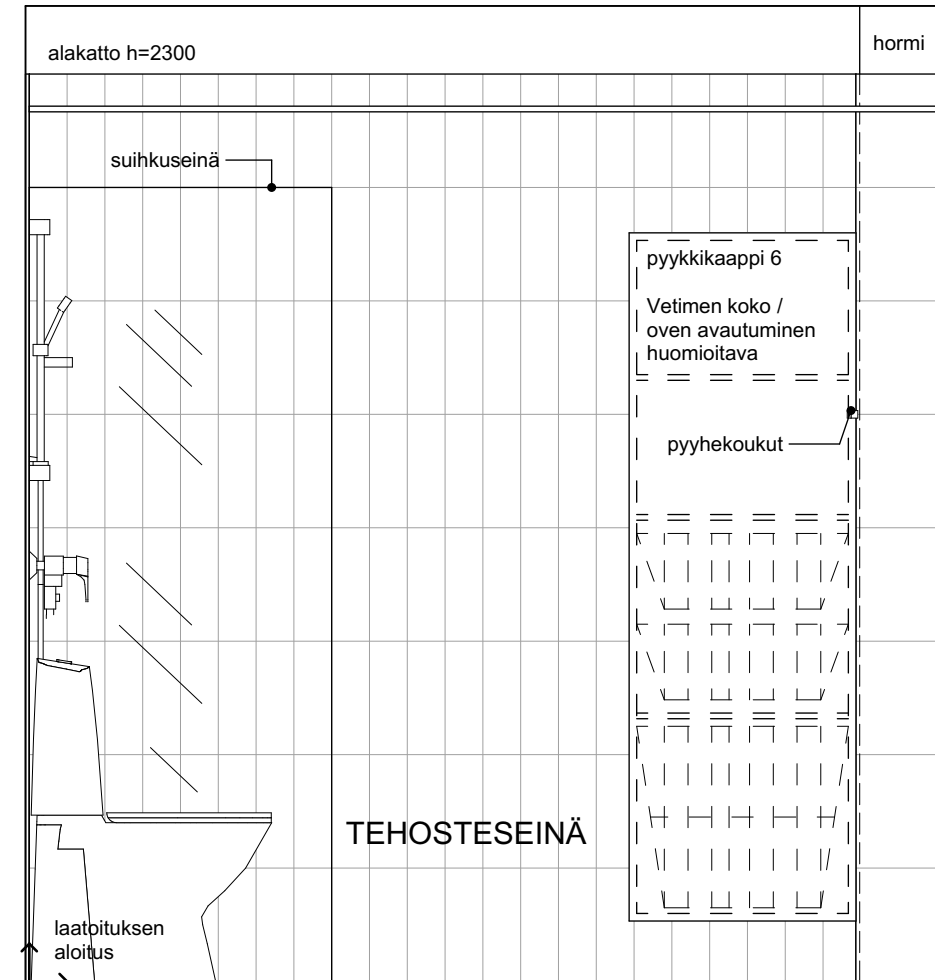
Saumat kohdakkain lattialaatoituksen saumojen kanssa!
