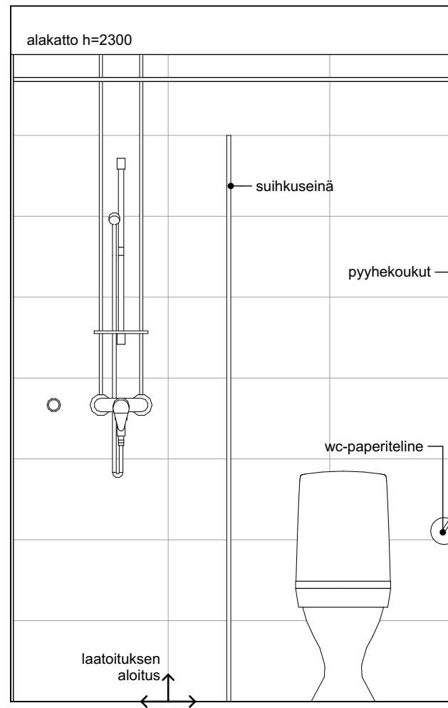
Saumot kohdakkain lattialaatoituksen saumojen kanssa!
